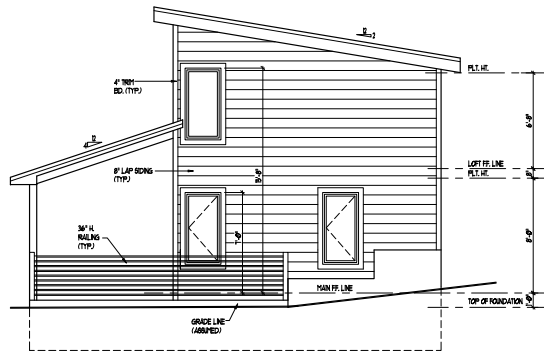
RIGHT ELEVATION SCALE: 1/4" = 1'-0"
